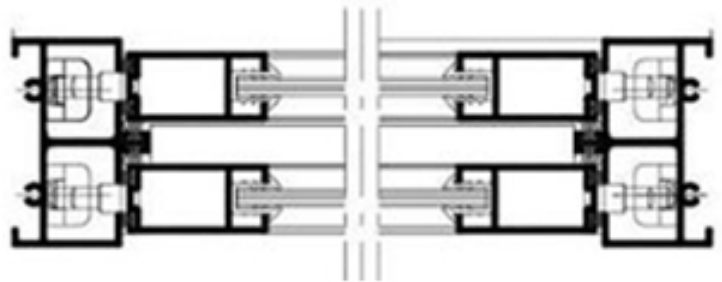
CORTE HORIZONTAL
